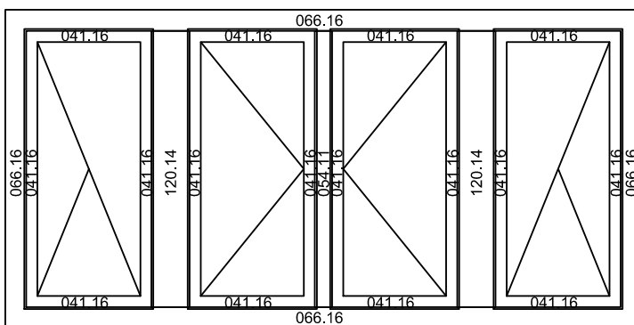
Typ 18) Fenster vierflügelig mit 2 Setzhölzern und einer Schlagleiste
